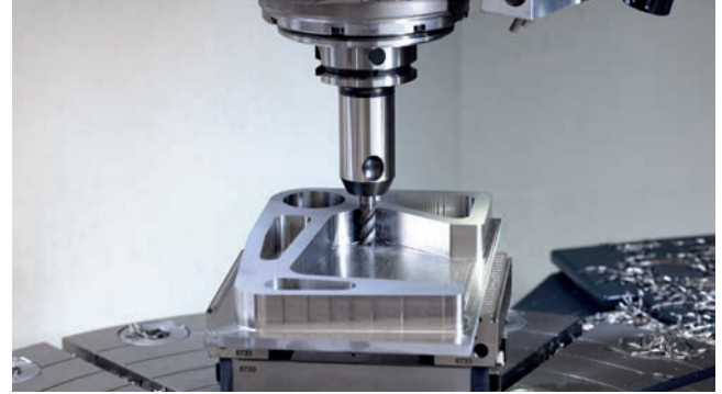
Werkzeug: VHM-Schaftfräser Ø 10 mm Werkstückmaterial: 1.4104
